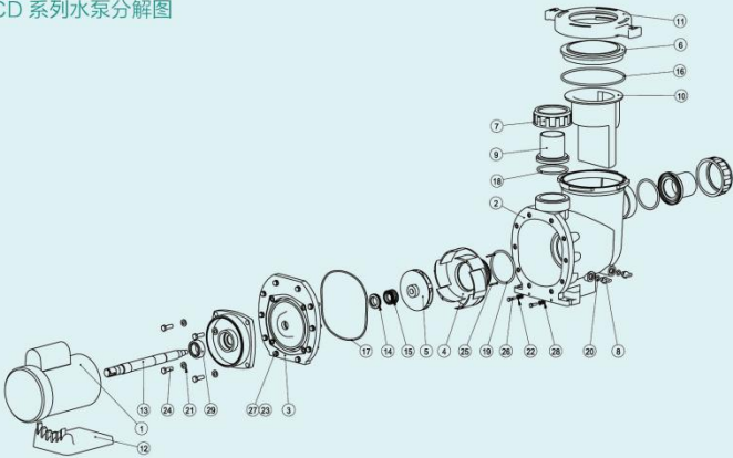
CD 系列水泵分解图
